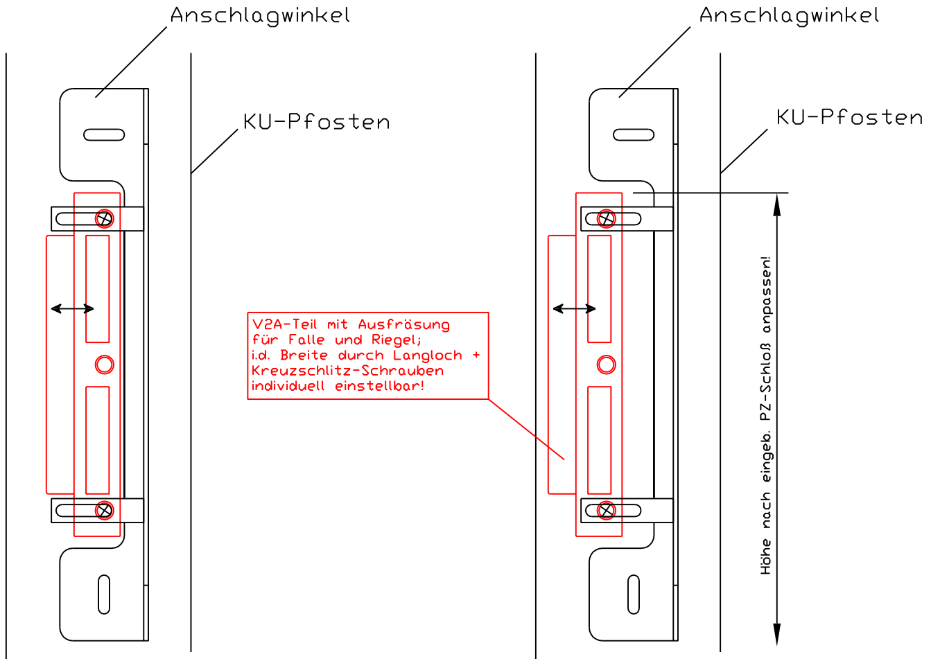
bei SS-Doppeltor (mit aufgedoppeltem Rahmen)
