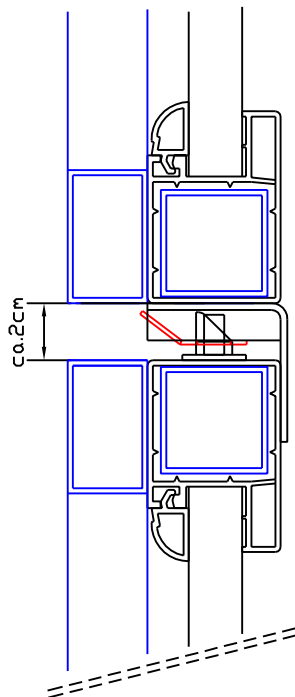
bei SS-Doppeltor (mit aufgedoppeltem Rahmen)
